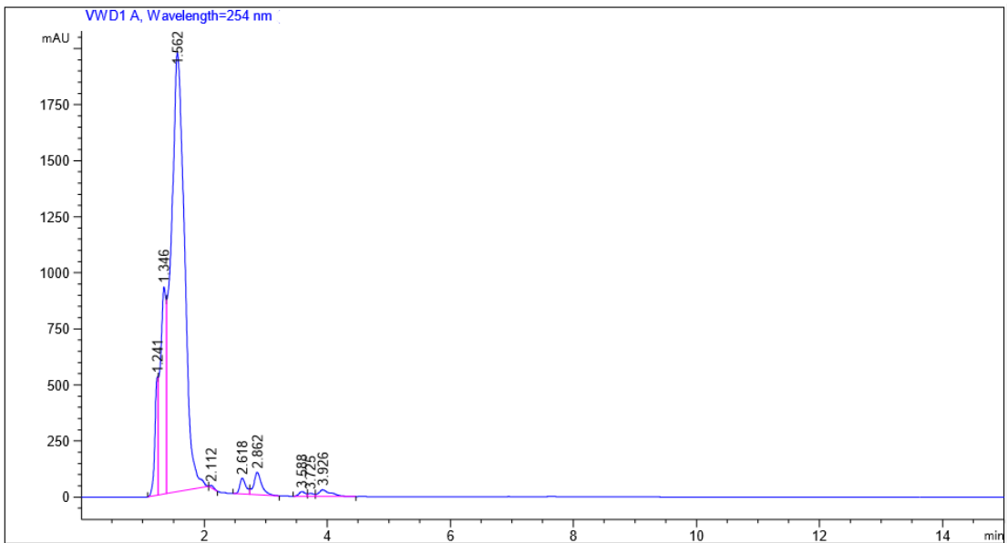
ภาพ ก-6 กราฟความสัมพันธ์ พื้นที่ และความเข้มข้น สกลนครตัวอย่างขึ้นงานที่ 6
