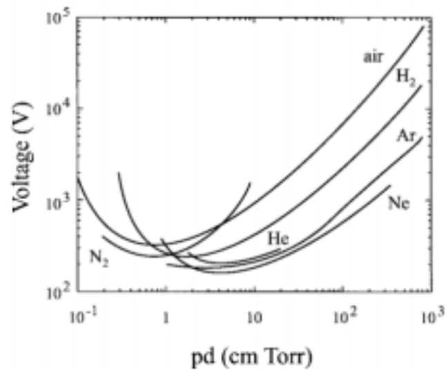
ภาพ 2.9 กราฟความสัมพันธ์ระหว่าง pd และ V_b ตามกฎของ Paschen ของก๊าซชนิดต่างๆ
