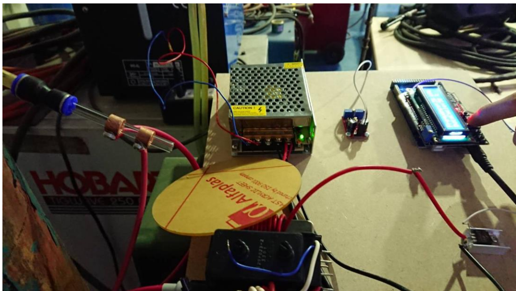
ภาพ 4.4 การต่อวงจรที่ใช้ในการทดลองครั้งที่ 1
