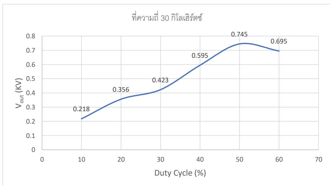
ภาพ 4.27 กราฟแนวโน้มของเปอร์เซ็นต์ดีวตี้ไซเคิลที่เหมาะสมที่ความถี่คงที่ 30 กิโลเฮิร์ตซ์
