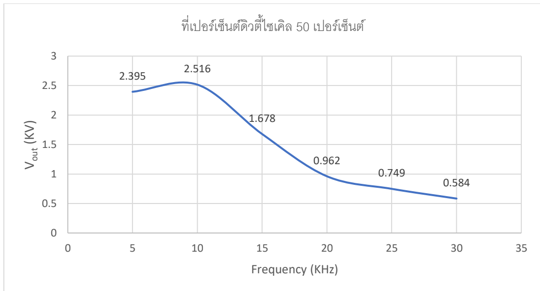
ภาพ 4.28 กราฟแนวโน้มของความถี่ที่เปอร์เซ็นต์ดีวีดีไซเคิลคงที่ 50 เปอร์เซ็นต์
