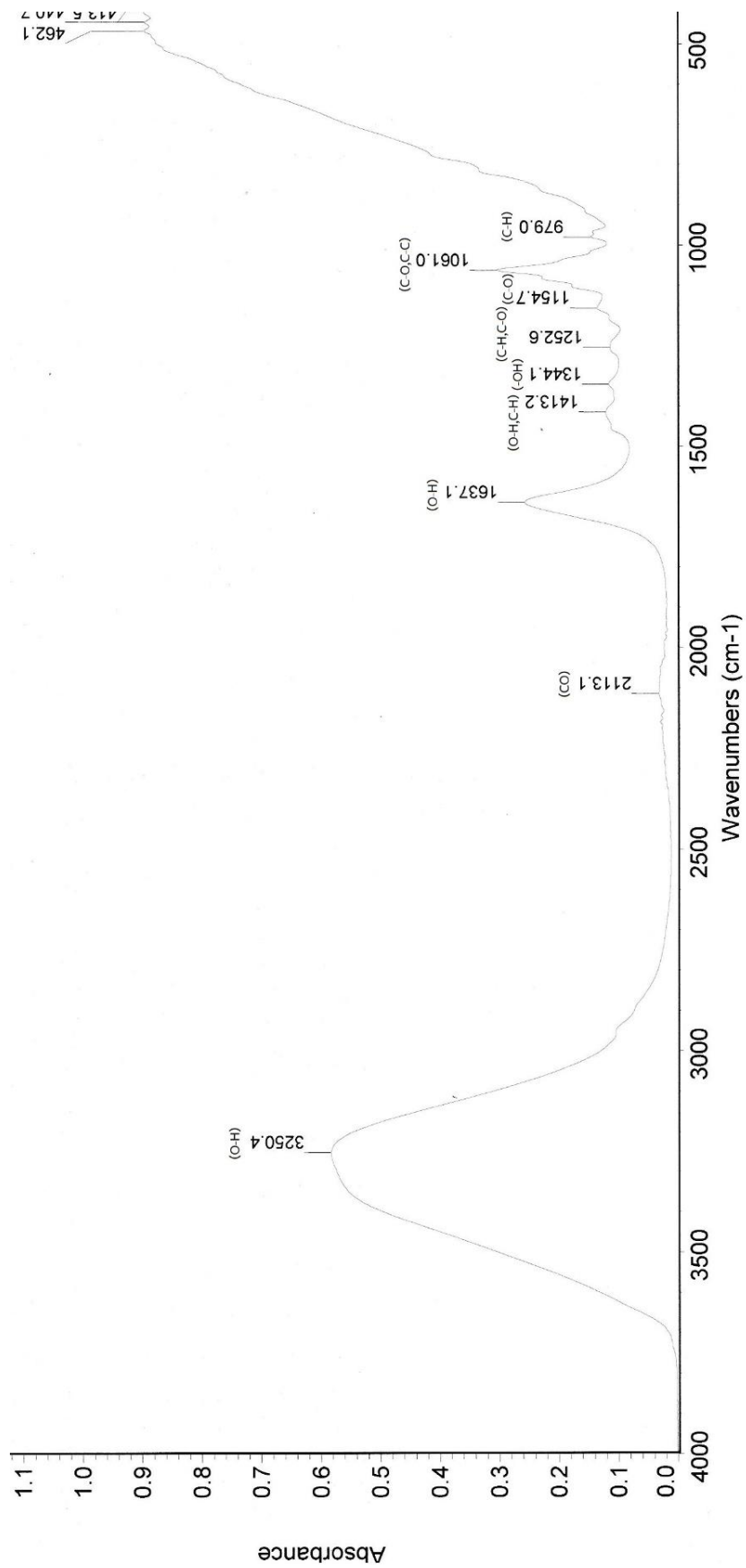
ภาพ ค-1 ผลทดสอบด้วยเครื่องนิวเคลียร์แมกเนติกเรโซแนนซ์สเปกโทรสโกปีของน้ำตาลฟรุคโตส ไฮโดรเจน
