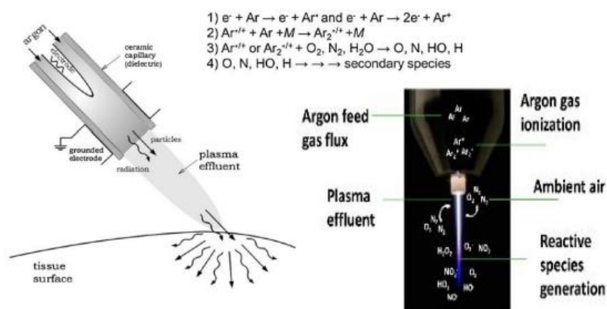
ภาพ 2.3 ปฏิกริยาที่เป็นไปได้เมื่อมีการเกิดการกระตุ้นของก๊าซอาร์กอนที่ทำให้เกิดอนุพันธ์ออกซิเจนที่ว่องไวและอนุพันธ์ไนโตรเจนที่ว่องไว
