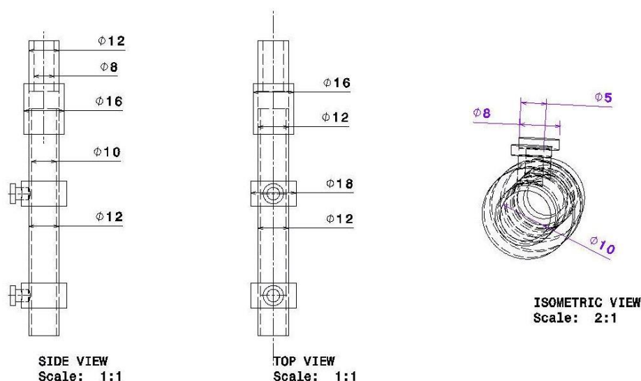
ภาพ 3.2 แบบจำลองโปรบิเล็กโทรดที่ทำการออกแบบ
