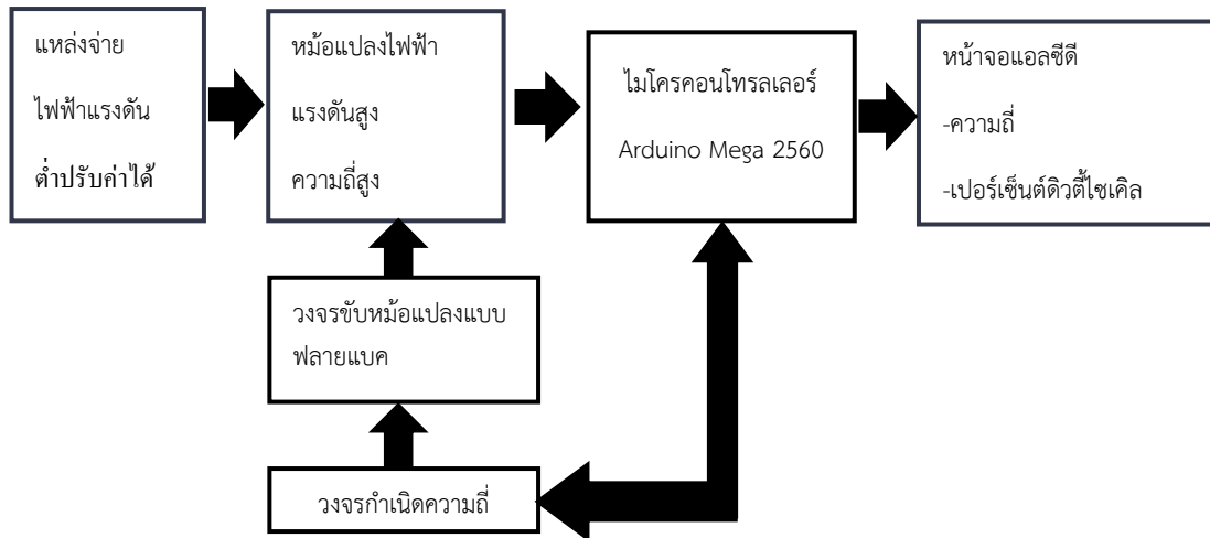
ภาพ 3.4 แบบโครงสร้างที่ใช้ในการประกอบแหล่งจ่ายไฟฟ้าแรงดันสูงความถี่สูงชนิดกระแสสลับ
