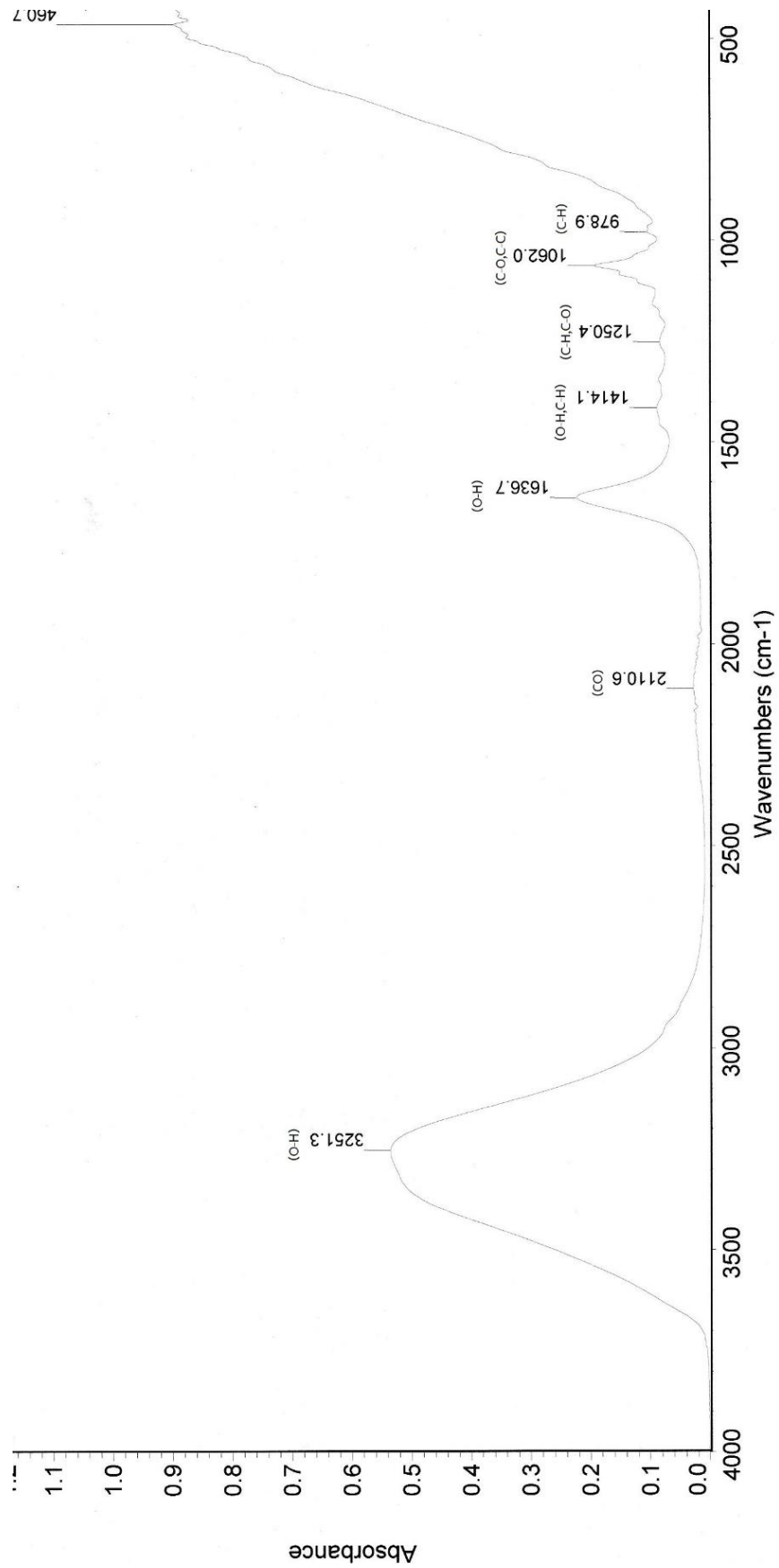
ภาพ ค-2 ผลทดสอบด้วยเครื่องนิวเคลียร์แมกเนติกเรโซแนนซ์สเปกโทรสโกปีของน้ำตาลฟรุกโตสไซรัปที่ได้ทำการดิสซอร์จ
