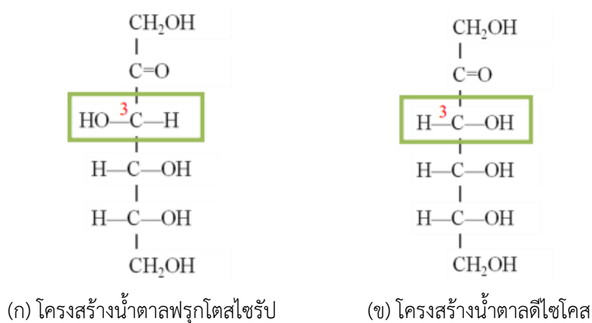
ภาพ 2.16 โครงสร้างน้ำตาลฟรุกโตสไซรัปและน้ำตาลหายาก (Rare Sugar) (ก) (ข)
