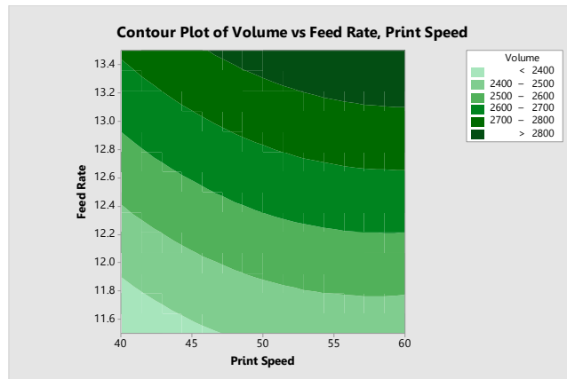
ภาพ 4.4 กราฟโครงร่างปริมาตร ระหว่างอัตราการพิมพ์และอัตราการฉีดขึ้นรูป
