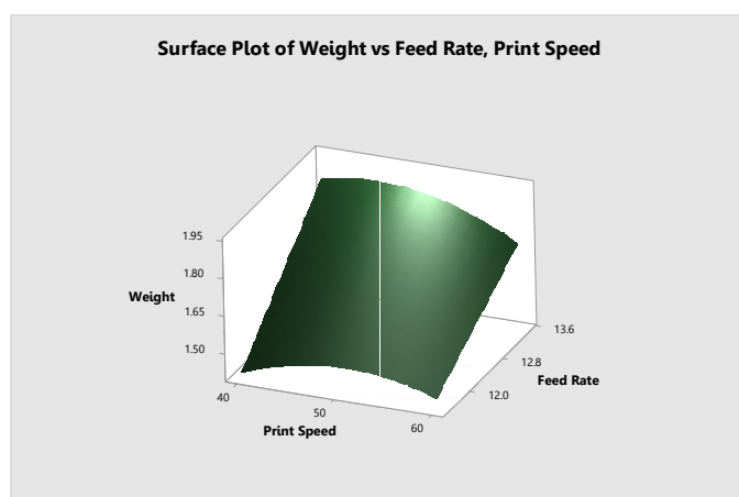
ภาพ 4.1 พื้นผิวผลตอบของน้ำหนักระหว่างอัตราการฉีดขึ้นรูปและอัตราเร็วการพิมพ์
