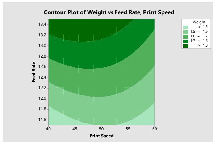
ภาพ 4.2 กราฟโครงร่างน้ำหนัก ระหว่างอัตราเร็วการพิมพ์และอัตราการฉีดขึ้นรูป
