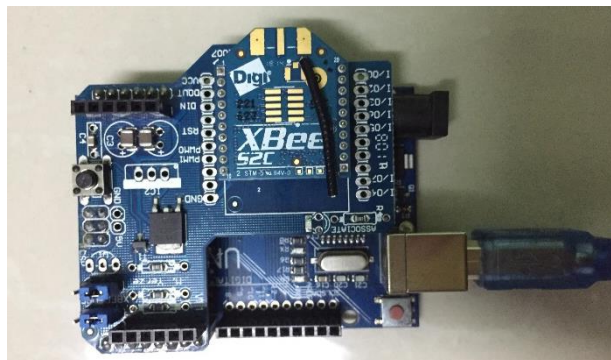
ภาพ 3.36 แสดงการเชื่อมต่อของอุปกรณ์กลุ่ม 2
