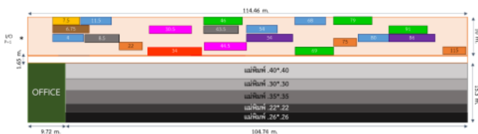
ภาพ 4.3 การวางสินค้าในคลังแบบไร้รูปแบบ (ก่อนปรับปรุง)
