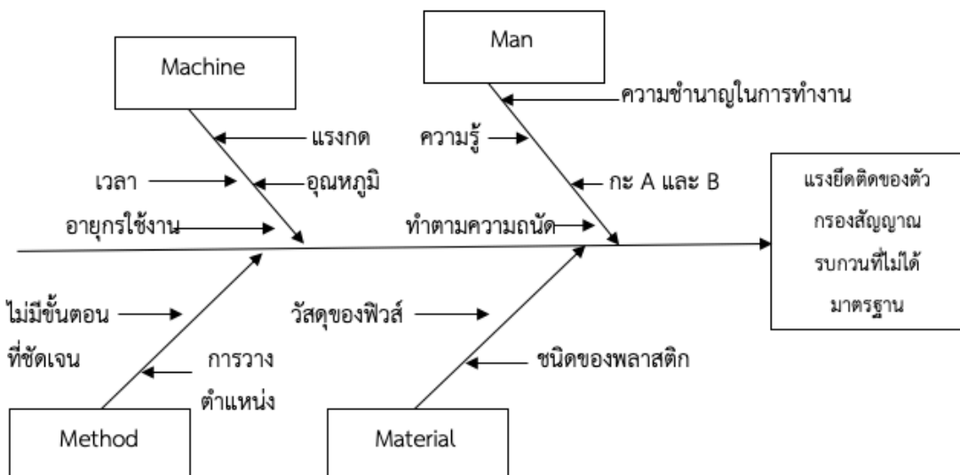
ภาพ 4.3 แผนผังก้างปลาแสดงสาเหตุที่ทำให้ปลั๊กและฟิวส์ยึดติดกันไม่ดี
