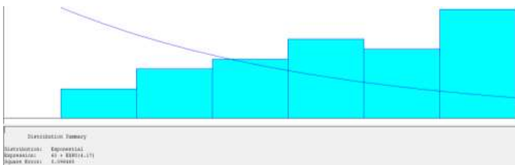
ภาพ ก-74 แสดงชนิดของการกระจายข้อมูลแบบมีรูปแบบนำเข้ากอง 1122
