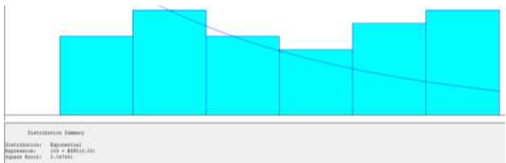
ภาพ ก-82 แสดงชนิดของการกระจายข้อมูลแบบไร้รูปแบบนำออกกอง 1035
