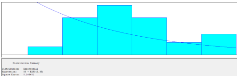
ภาพ ก-79 แสดงชนิดของการกระจายข้อมูลแบบไร้รูปแบบนำออกกอง 1030
