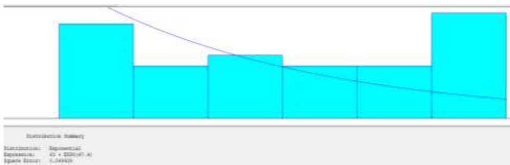
ภาพ ก-57 แสดงชนิดของการกระจายข้อมูลแบบมีรูปแบบนำเข้ากอง 1122
